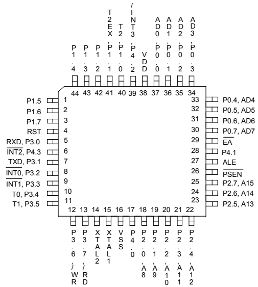
44-Pin QFP (W78E65F)
