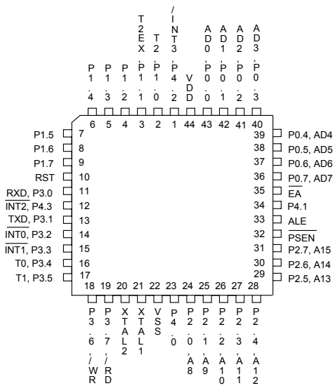
44-Pin PLCC (W78E65P)
